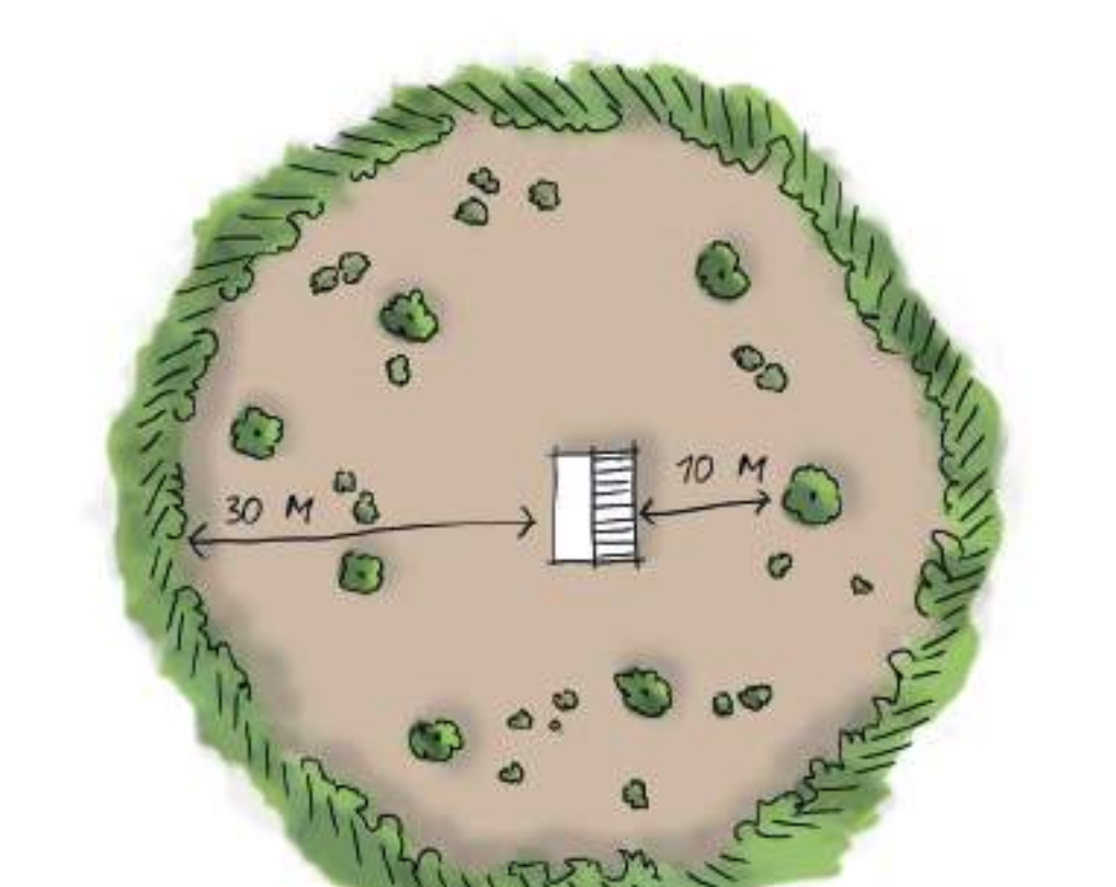
BOVENAANZICHT REGELS BRANDVEILIGHEID RONDOM VAKANTIEWONINGEN
